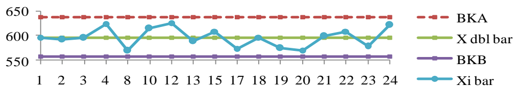
Gambar 2 Grafik Batas Kontrol
