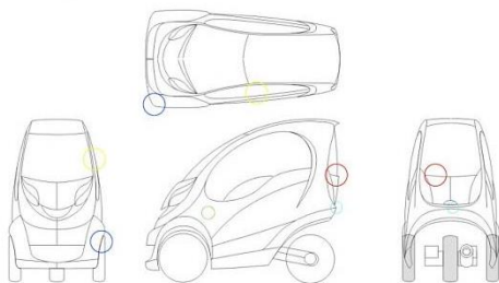
Gambar 16 Revisi Pertama
