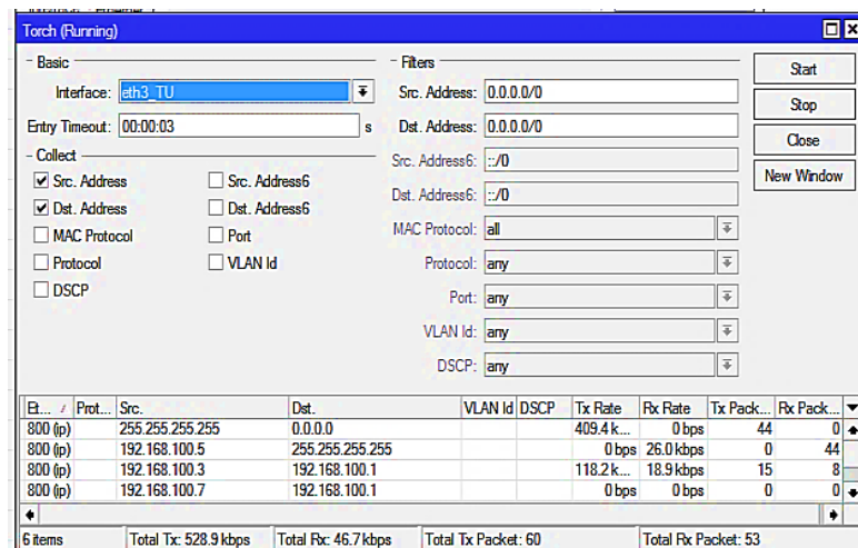
Gambar 12 Torch Mikrotik
