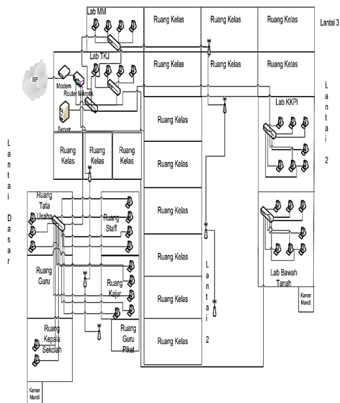
Gambar 2 Rancangan topologi physical setelah terpasang Router Mikrotik
