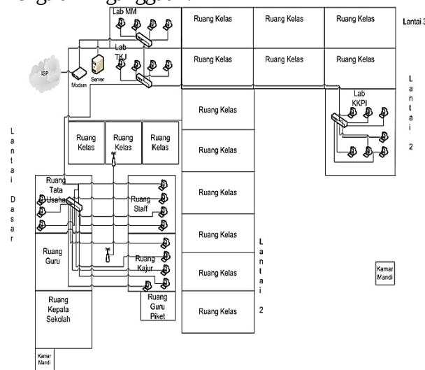
Gambar 1 Topologi physical yang sedang terpasang
